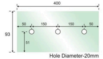
DFP-400 Fin Plate 400mm
